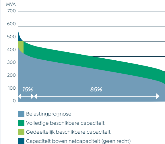
Inpassingsvoorbeeld o.b.v. belastingduurkromme
